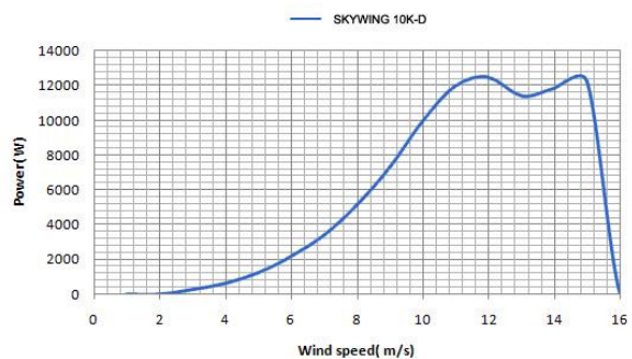
(10 kW võrgulahendusega elektrituulik Eestis 02.2012)
